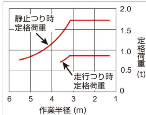
定格荷重曲線
