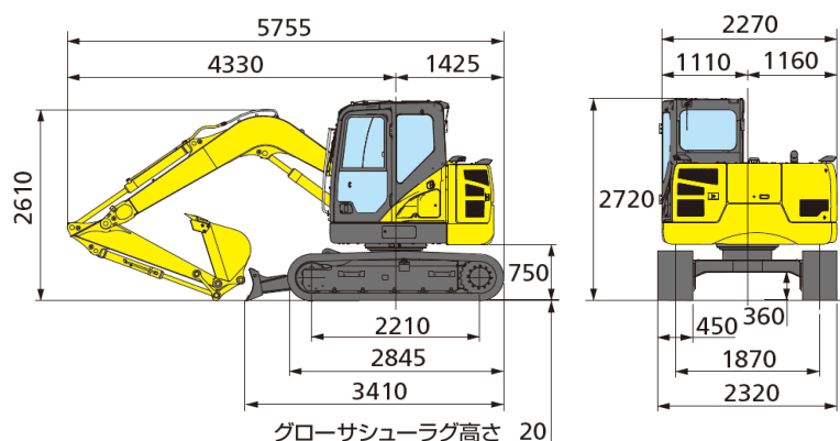
■ 寸法図
