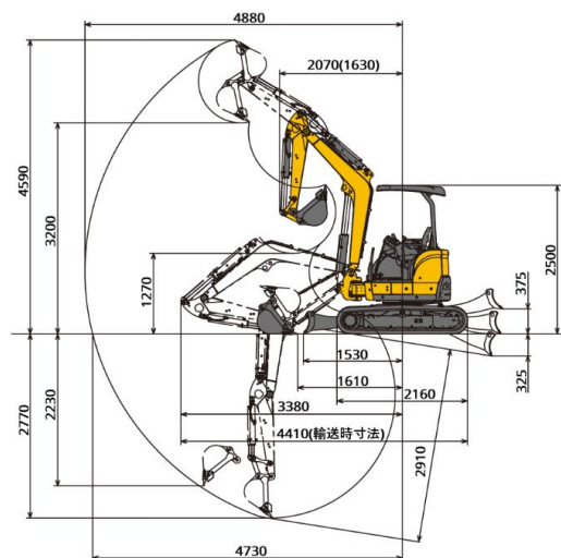
■作業範囲図(単位:mm)
