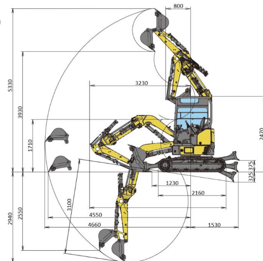
■作業範囲図(単位:mm)
