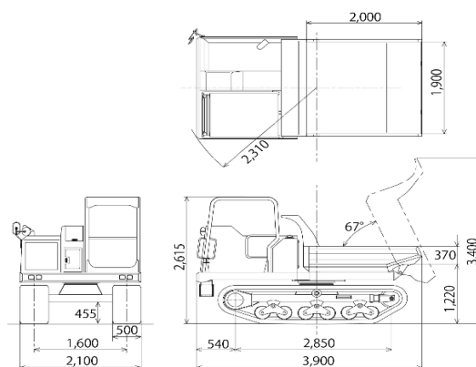
本体寸法図 mm
