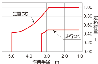
■ クレーン定格荷重曲線
