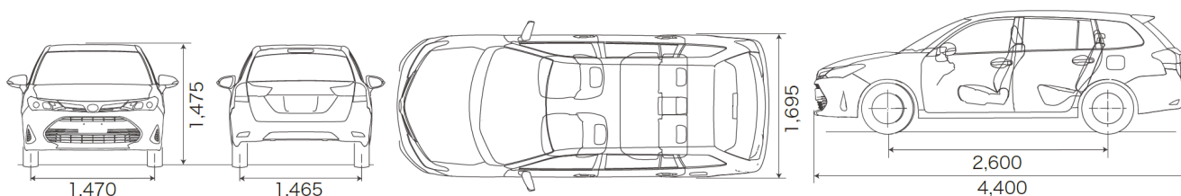
■寸法図 単位: mm
