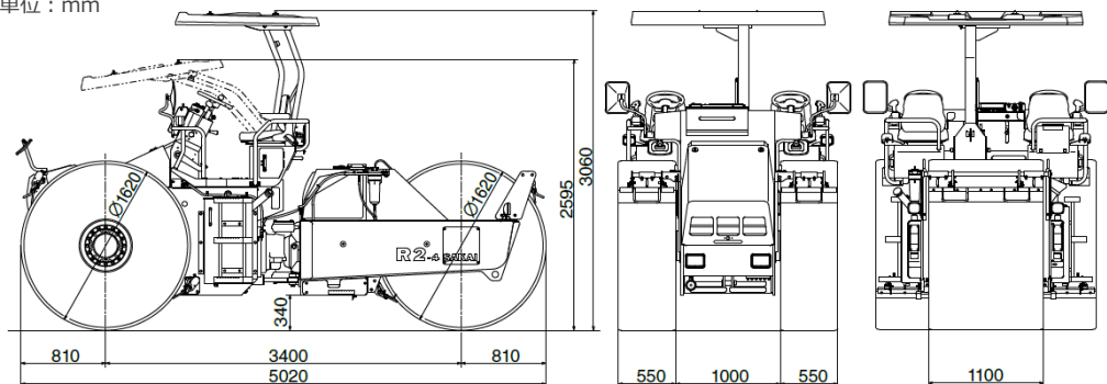
■寸法図 単位：mm
