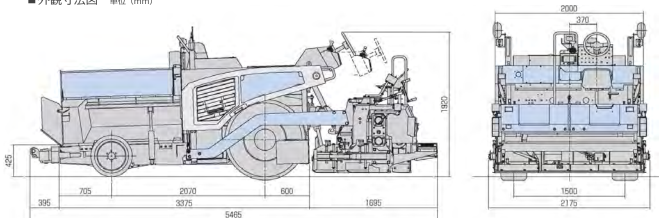
■外観寸法図 単位 (mm)
