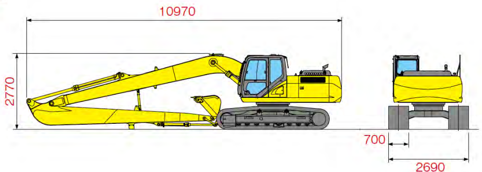
●外観寸法図 単位 (mm)
