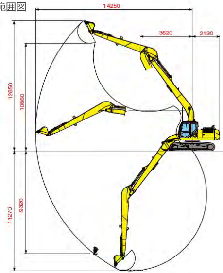
●作業範囲図
