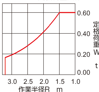
■クレーン定格荷重曲線
