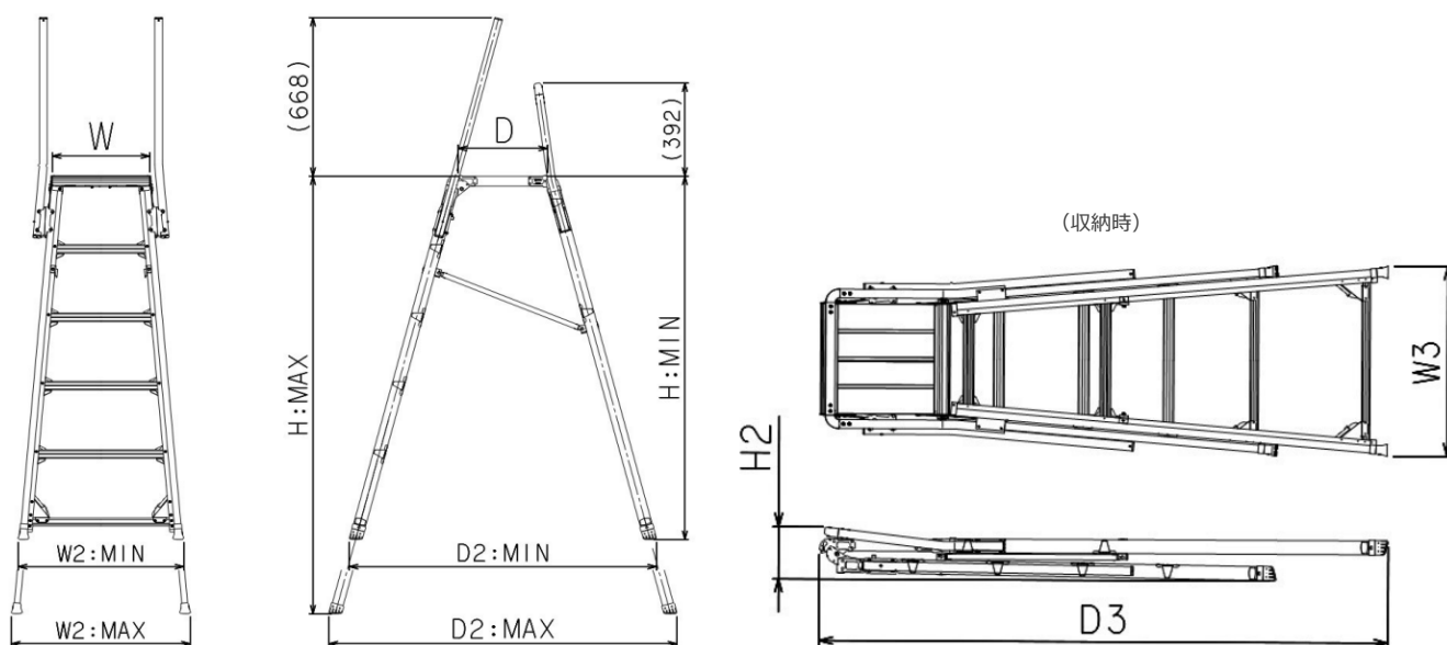
■寸法図 単位 : mm
