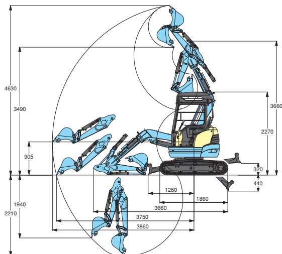
●作業範囲図 単位 (mm)
