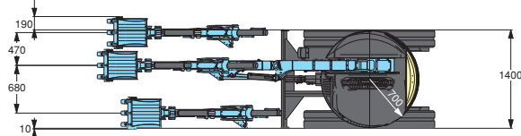
●外形寸法図 単位 (mm)
